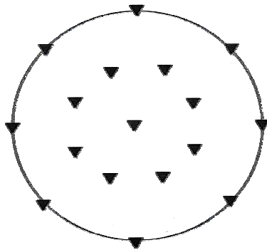
Figuur A.1: aantal sonderingen voor tanks met een diameter tussen 25 en 50 m
