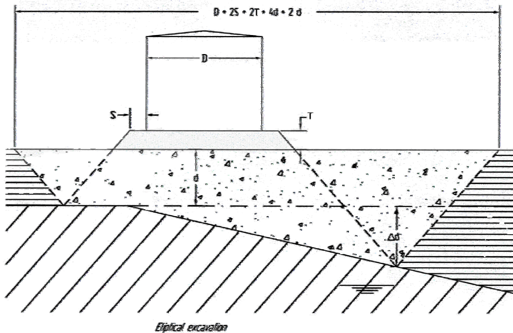
Figuur A.4: grondverbetering op ongelijk niveau
